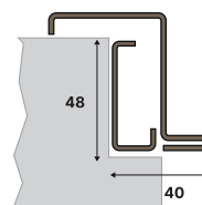
Premarco superreducido y marco reducido
