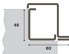
Premarco y marco reducidos
