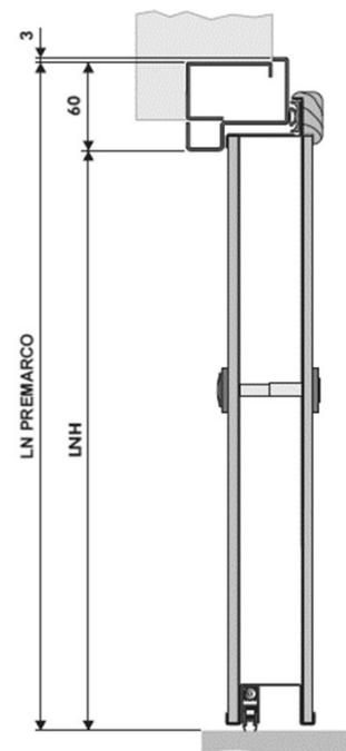
Sección vertical:
